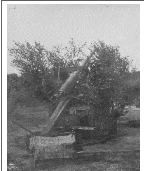
Mont Ganelon, fin 1915 : pièce de 75 anti-aérienne fixée sur plateforme et camouflée par des branches d'arbre. Cette plate-forme du modèle 1915 permet un tir à 360° sur une inclinaison de 0 à 75° (collection personnelle).
